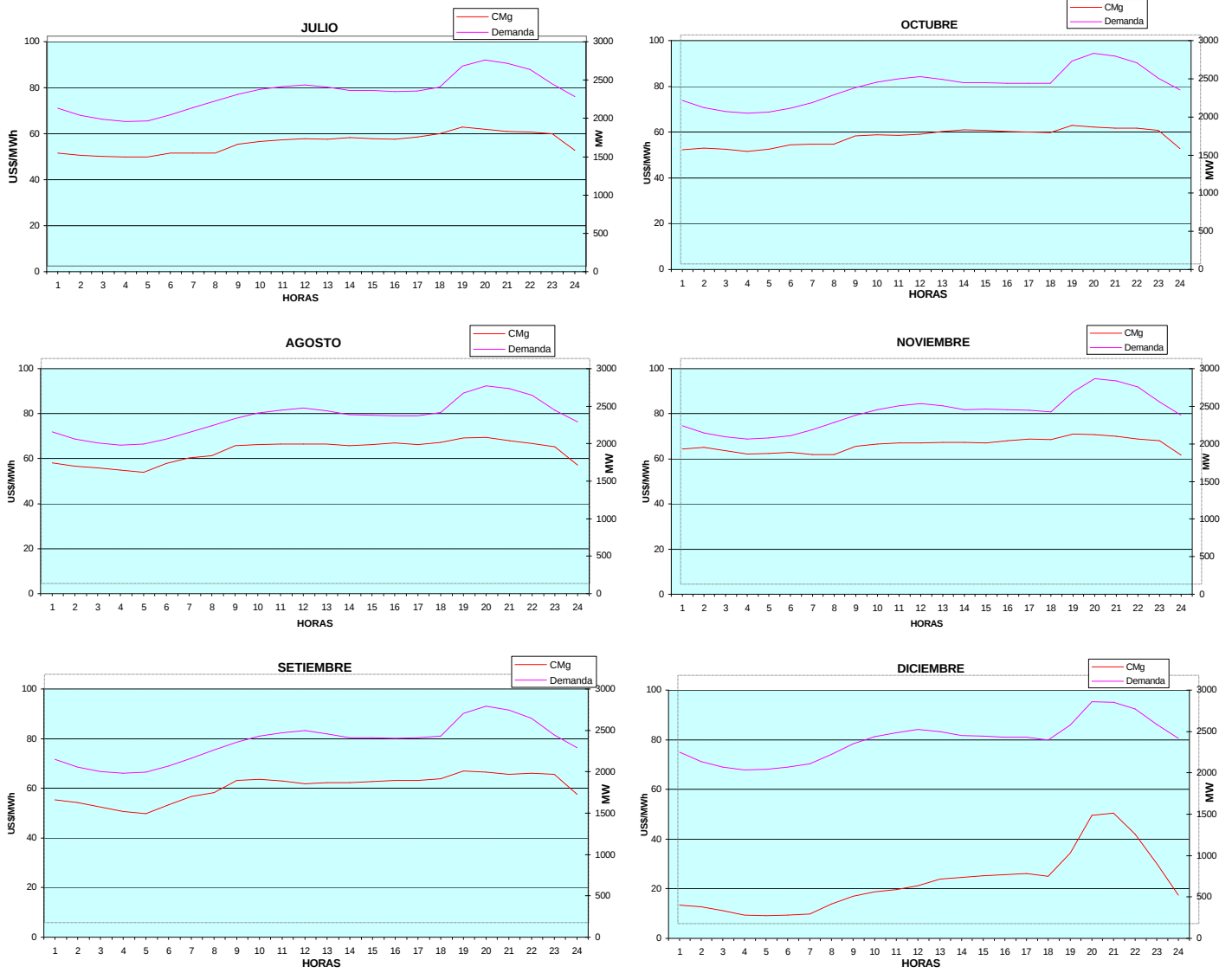
GRAFICO N° 7.5 COSTOS MARGINALES PROMEDIO HORARIO VS DEMANDA HORARIA PROMEDIO DEL MES SEIN 2003
