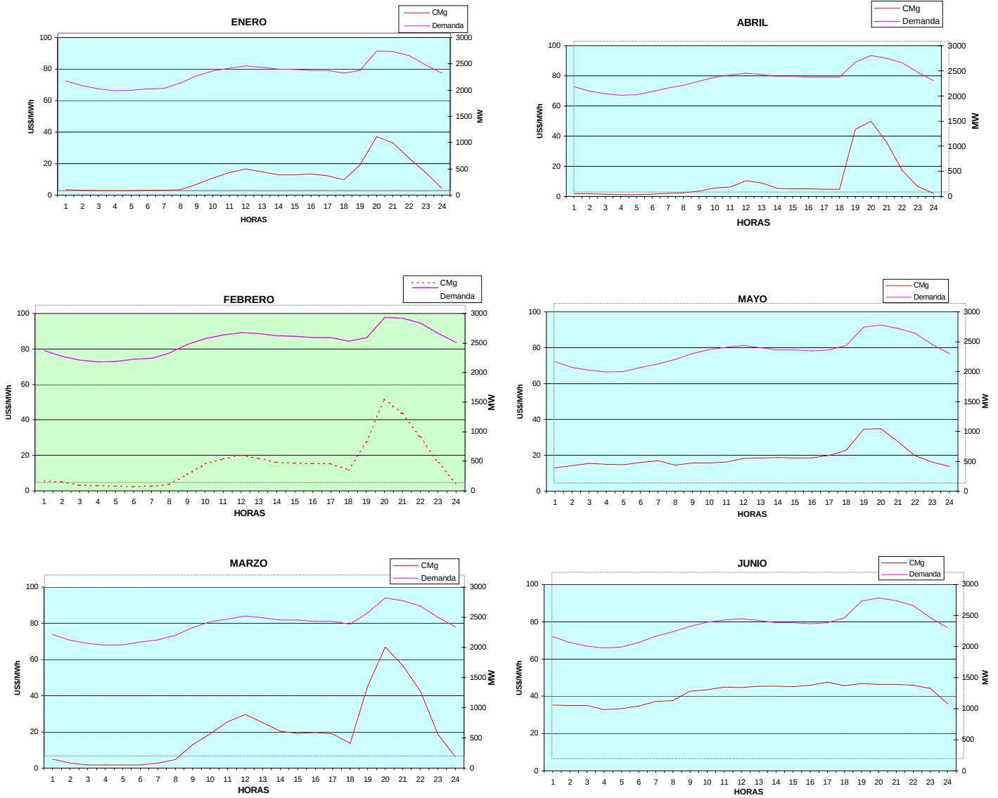
GRAFICO N° 7.4 COSTOS MARGINALES PROMEDIO HORARIO VS. DEMANDA HORARIA PROMEDIO DEL MES SEIN 2003
