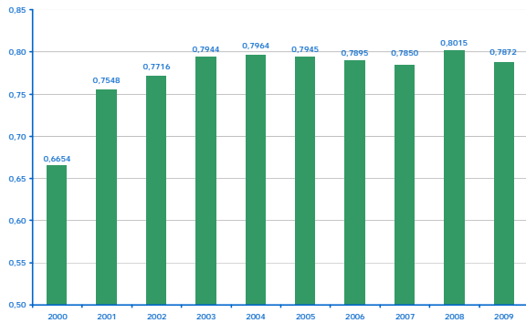
GRÁFICO N° 3.1 FACTORES DE CARGA DEL SEIN 2000 - 2009
