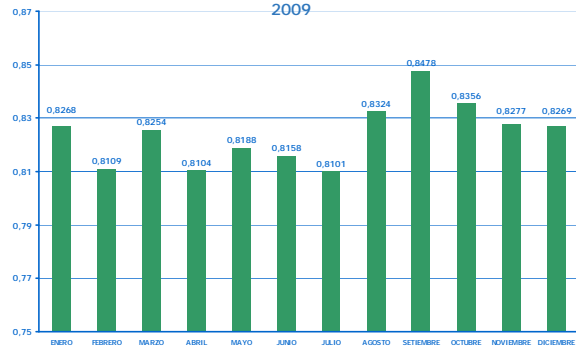
GRÁFICO N° 3.5 DIAGRAMA DE DURACIÓN MENSUAL DEL SEIN 2009
