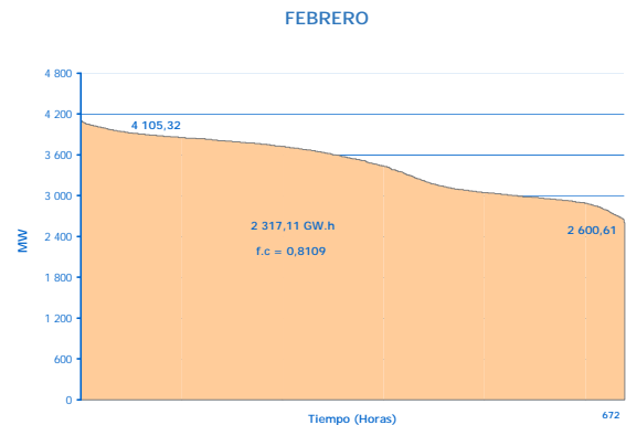
GRÁFICO N° 3.5 DIAGRAMA DE DURACIÓN MENSUAL DEL SEIN 2009
