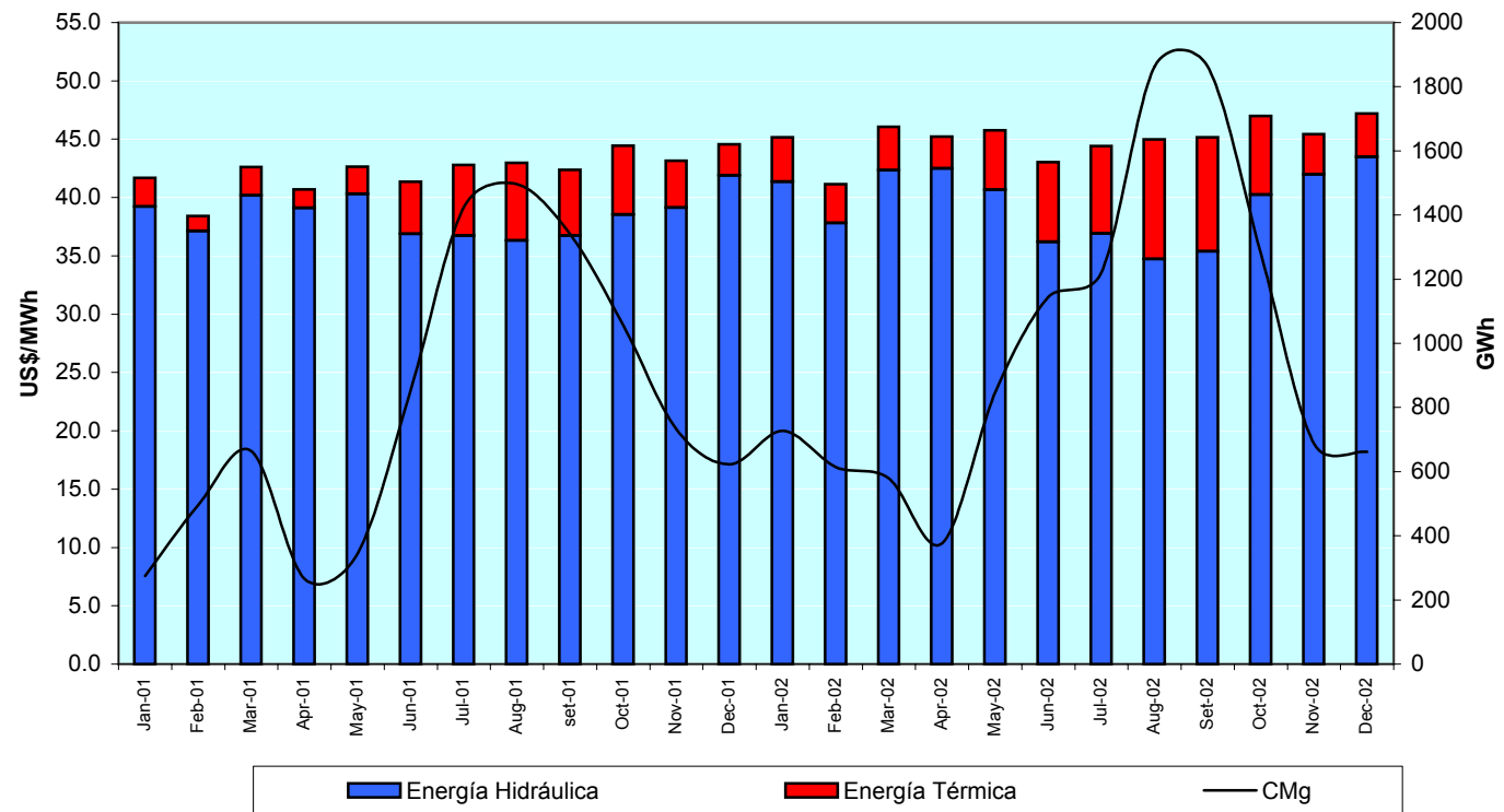
GRAFICO N° 7.6 Generación de energía mensual vs. Costos Marginales Promedio mensual
