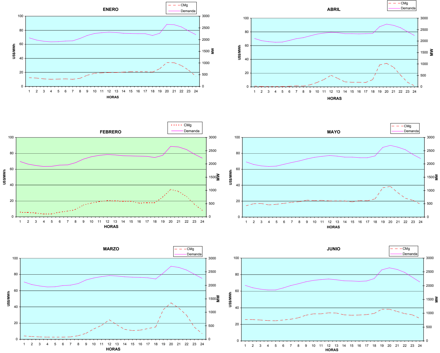
GRAFICO N° 7.4 COSTOS MARGINALES PROMEDIO HORARIO VS. DEMANDA HORARIA PROMEDIO DEL MES SINAC- 2002
