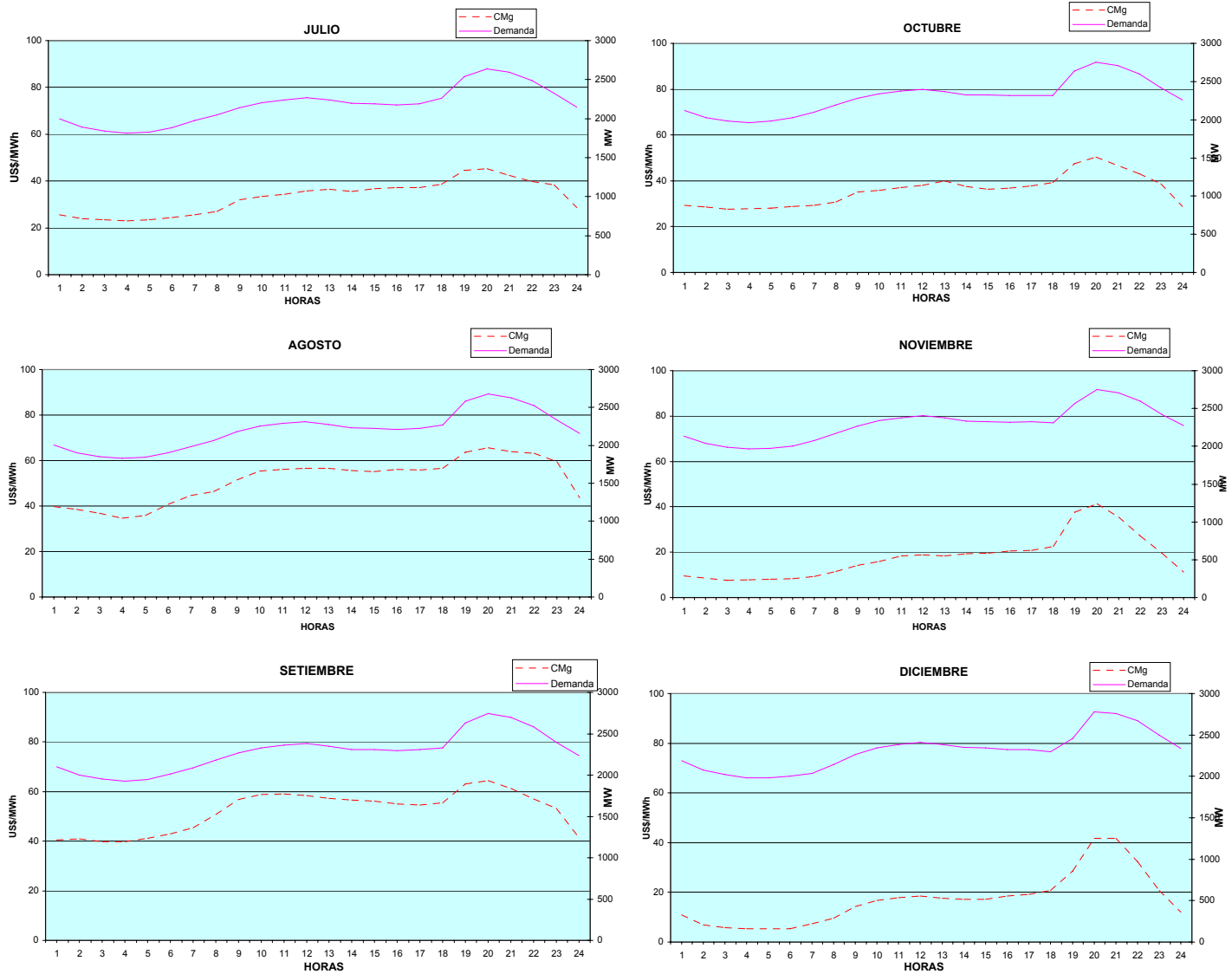
GRAFICO N° 7.5 COSTOS MARGINALES PROMEDIO HORARIO VS DEMANDA HORARIA PROMEDIO DEL MES SINAC - 2002
