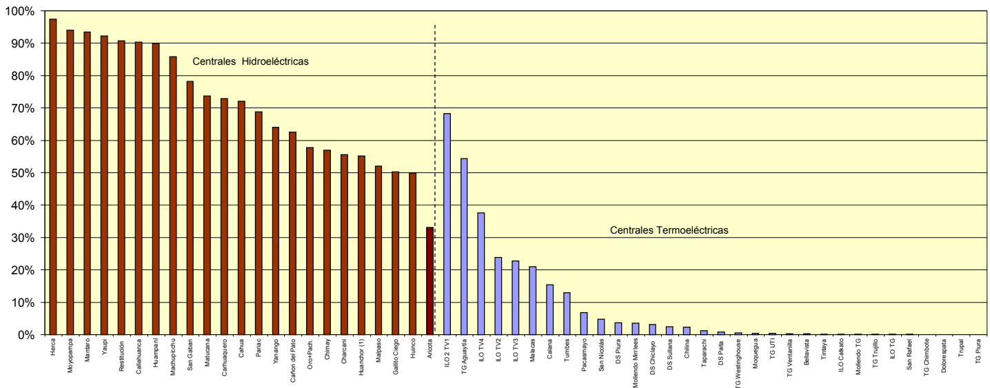
CENTRALES ELECTRICAS DEL SINAC ( Enero - Diciembre 2002 ) Factor de Planta Anual de Centrales
